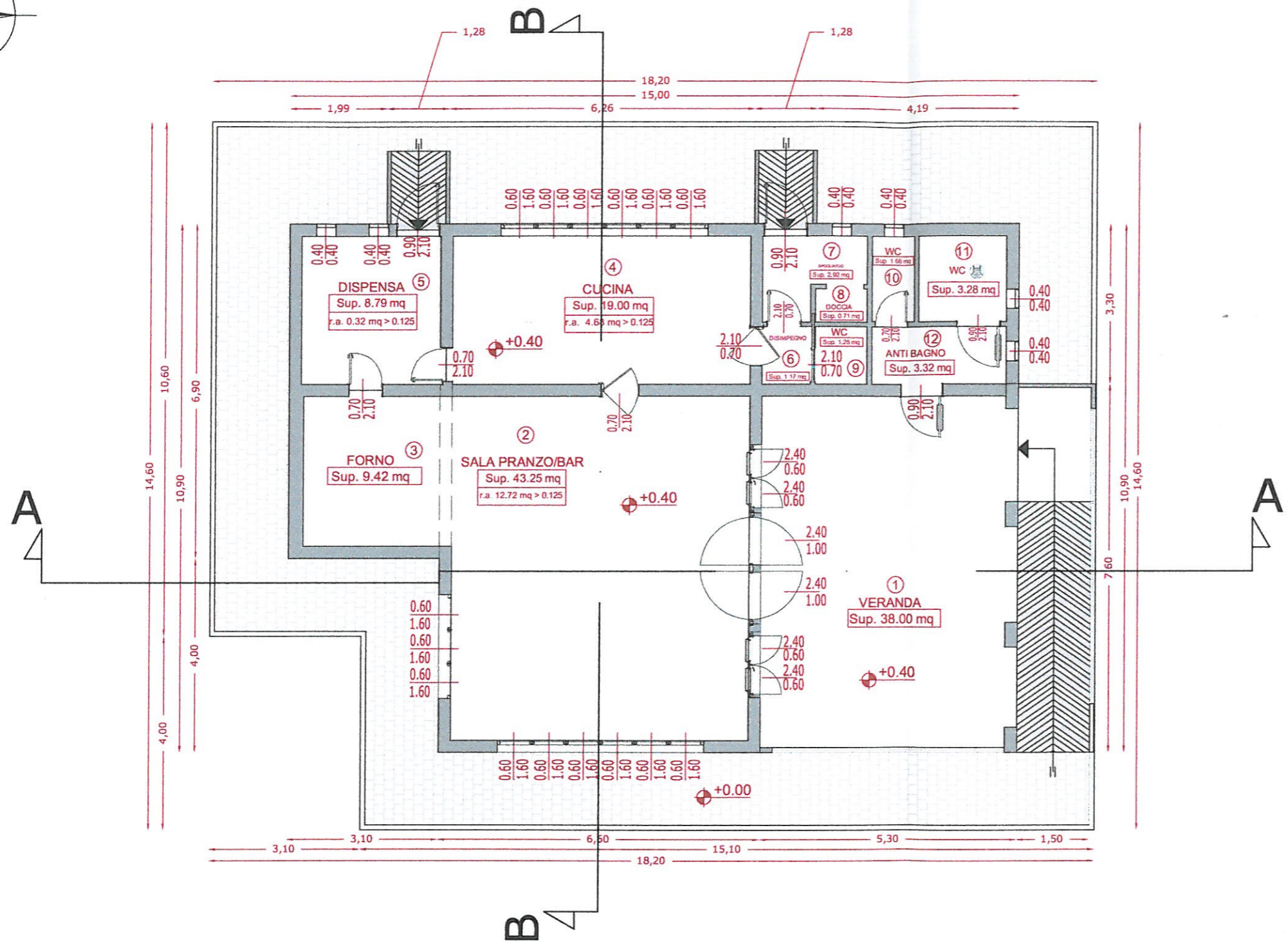
PIANTA PIANO TERRENO (quota + 0.40)
